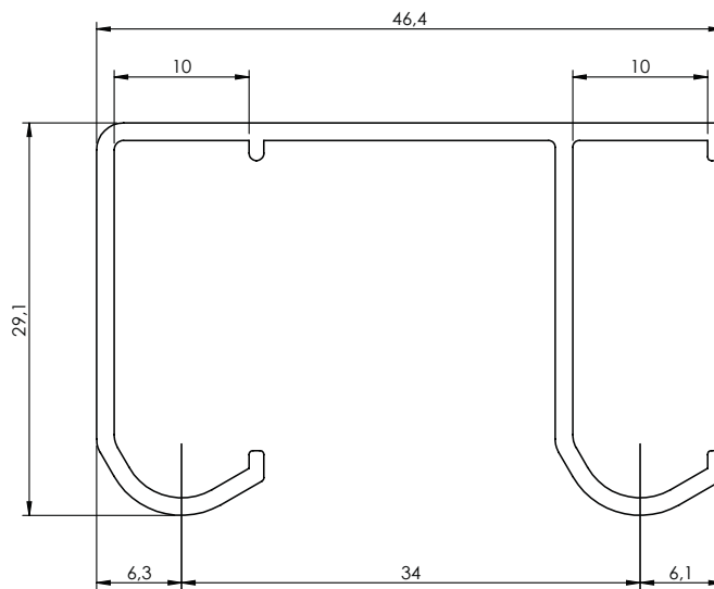
Obere Laufschiene
