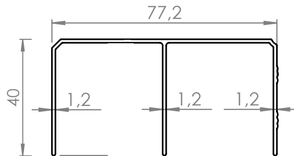
Deckenschiene, zweiläufig
