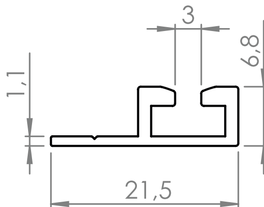
Bodenschiene, einläufig
