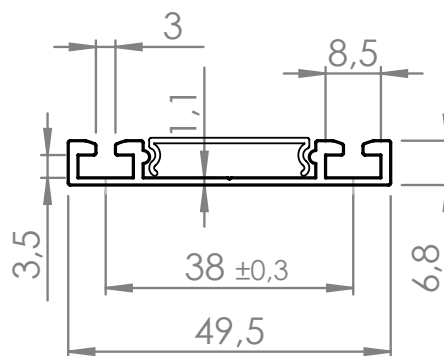
Bodenschiene, zweiläufig
