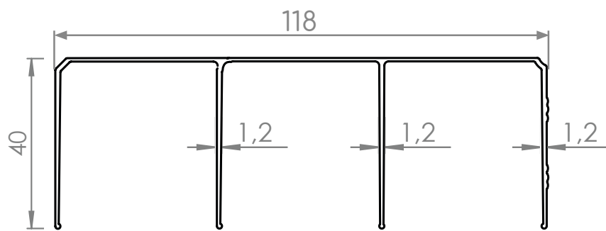
Deckenschiene, dreiläufig
