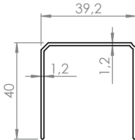
Deckenschiene, einläufig
